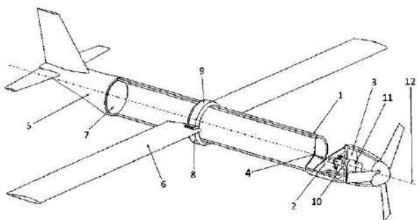
Samolot do prowadzenia obserwacji w stratosferze – Instytut Lotnictwa
